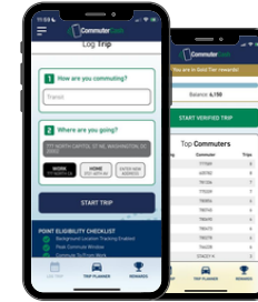
CommuterCash goDMV
